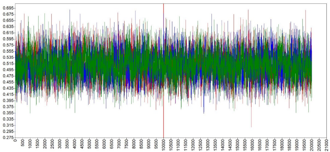
\text{Var}(e_Y)
