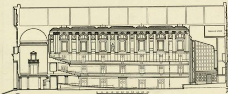
LONGITUDINAL SECTION
