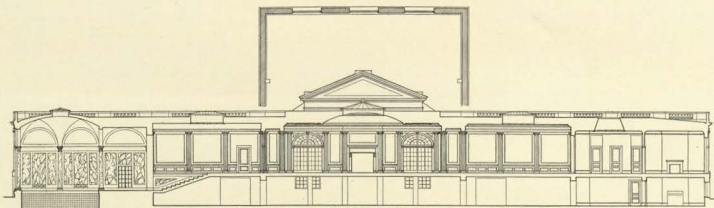
LONGITUDINAL SECTION
