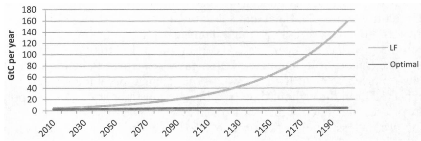
FIGURE 4.—Coal use: optimum versus laissez-faire.
