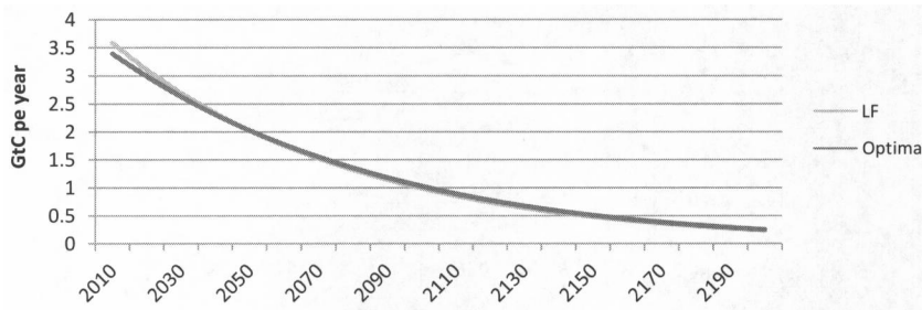
FIGURE 5.—Oil use: optimum versus laissez-faire.
